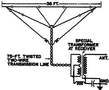
Spider-web antenna.
